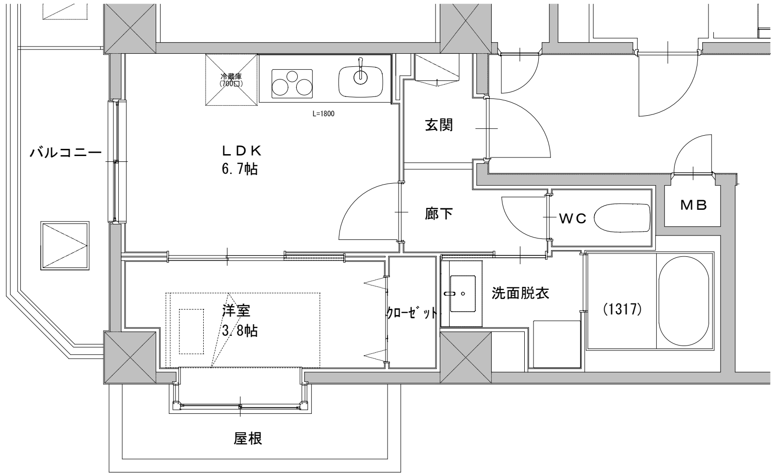
5階Nタイプ 床面積 31.36㎡
